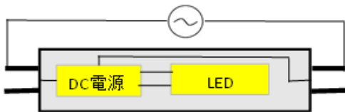
(蛍光灯内部配線図)
